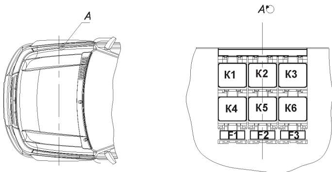
Рис. 2. Реле и предохранители:
